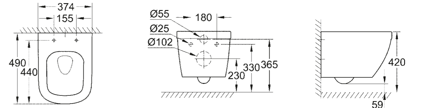
39 206 000 39 206 00H* Compact wall hung WC rimless
