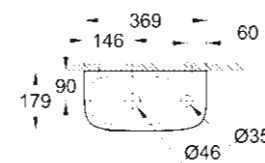
39 327 000 39 327 00H* Mini handrinse basin 37 cm
