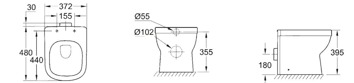
39 329 000 39 329 00H* Floorstanding WC rimless
