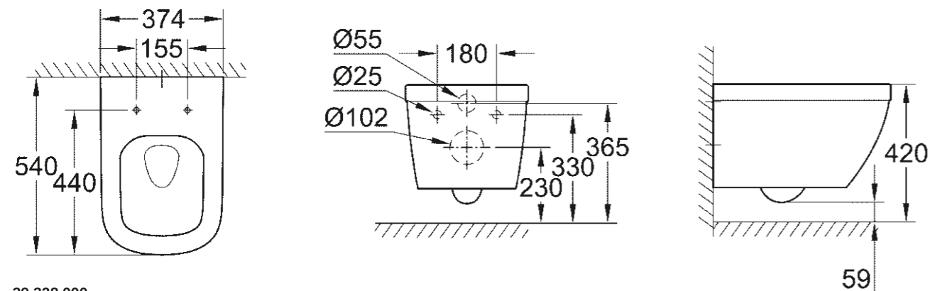
39 328 000 39 328 00H* Wall hung WC rimless
