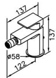
6790-99-81CP Bidet Mixer
