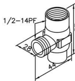
6790-TB-80CR Diverter
