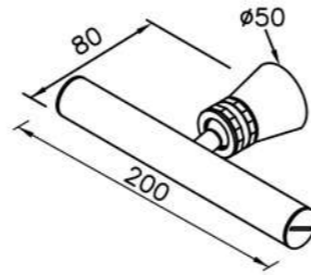
6874-AB-80CP Showerhead
