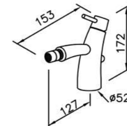
6780-99-81CP Bidet Mixer
