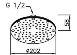
6771-AC-80CP 8" Showerhead
