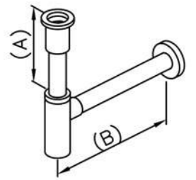
T-Trap 6502-TT-80CP A:170 B:340(mm) 6502-TT-81CP A:170 B:465(mm)
