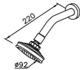
6803-AH-80CP Showerhead
