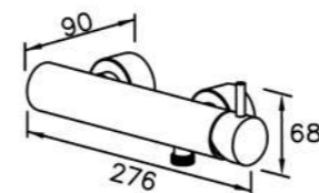
6771-93-80CP Shower Mixer Body
