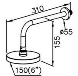
6771-AH-80CP 6" Showerhead
