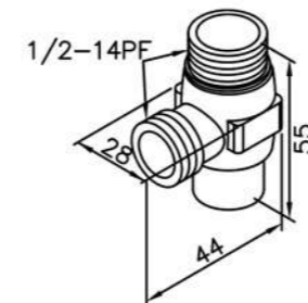
6790-TA-80CR Diverter
