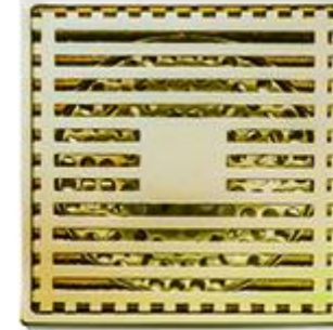
کفشوی برنجی ( کروم ) Size 100*100 mm Code 0303-64-79CP
