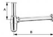
Bottle-Trap 6512-BT-80CP A:108 B:210 mm 6512-BT-81CP A:108 B:420 mm 6512-BL-80CP A:185 B:210 mm 6512-BL-81CP A:185 B:420 mm
