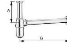
Bottle-Trap 6512-BT-80CP A:108 B:210 mm 6512-BT-81CP A:108 B:420 mm 6512-BL-80CP A:185 B:210 mm 6512-BL-81CP A:185 B:420 mm
