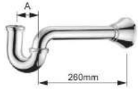
P-Trap 6122-A3-80CP A:73mm 1 1/2" 6122-B3-80CP A:65mm 1 1/4"
